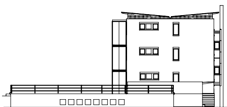
Anblick Süd
