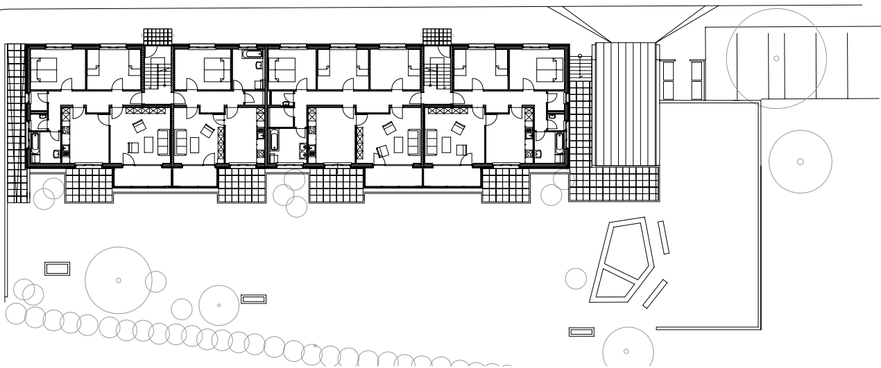
Erdgeschoss
